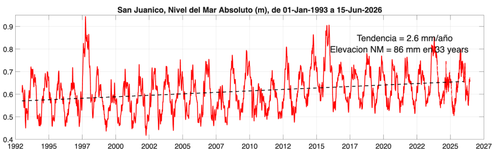
Figura 2.5: Nivel del mar absoluto (m) en la San Juanico, BCS, costa pacífico norte de BCS. Inicia en enero de 1993 y termina en junio de 2026. Incluye el nivel del mar con referencia al geoide y la tendencia de largo período debida al calentamiento global. Este sitio representa la variabilidad del Golfo de Ulloa.
