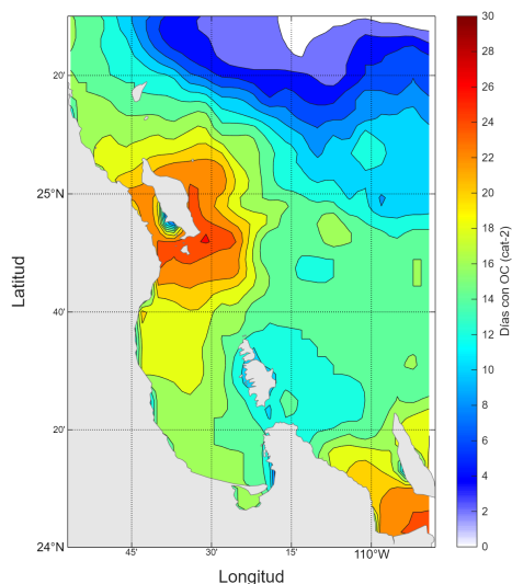
Figura 5.9: Cantidad de días con ondas de calor categoría 2 para la región comprendida entre Isla Cerralvo a isla San José, incluyendo la bahía de La Paz.
