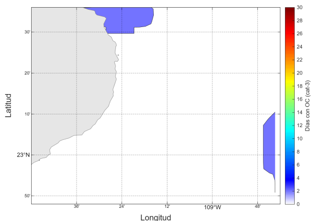
Figura 5.7: Cantidad con días con ondas de calor de categoría 3 en Cabo Pulmo y zonas aledañas para mayo de 2026.
