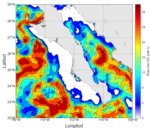
Figura 5.1: Días con ondas de calor categoría 1 en el área de estudio para mayo de 2026.
