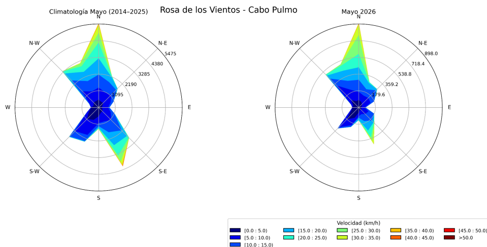
Figura 8.2: Climatología vs. observaciones de la dirección e intensidad de los vientos en la estación Cabo Pulmo durante el mes de mayo de 2026.
