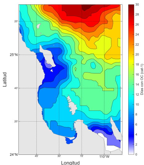
Figura 5.8: Cantidad de días con ondas de calor categoría 1 para la región comprendida entre Isla Cerralvo a isla San José, incluyendo la bahía de La Paz.
