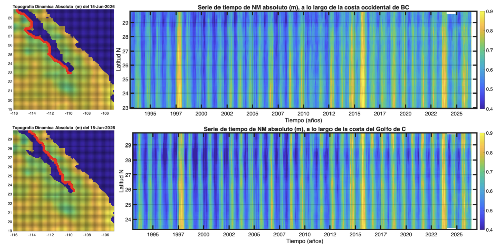
Figura 2.1: Evolución del nivel del mar (NM absoluto) a lo largo de las dos costas de la península de BC desde enero de 1993 hasta junio de 2026. Arriba: costa occidental; abajo: costa del Golfo de California.
