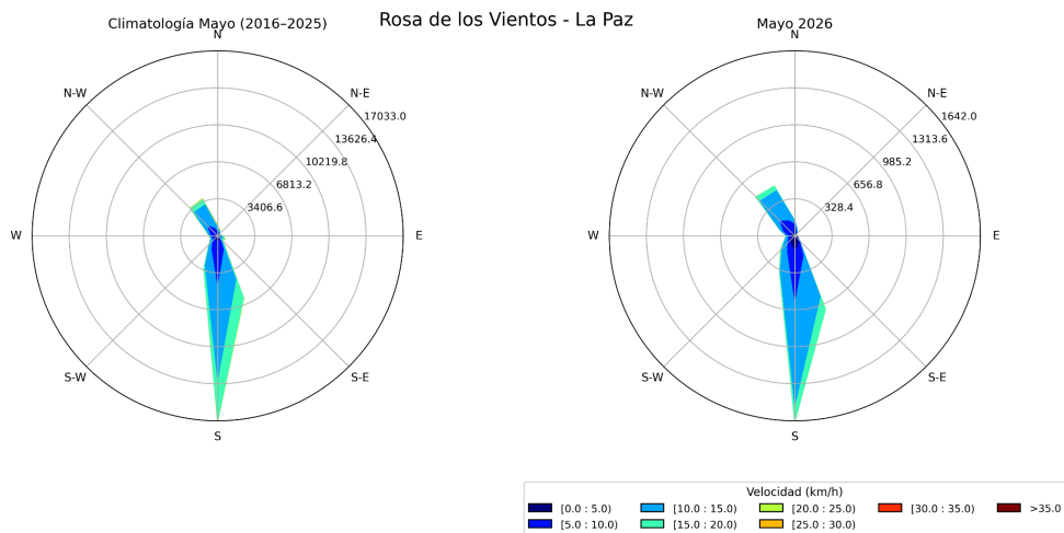
Figura 8.4: Climatología vs. observaciones de la dirección e intensidad de los vientos en la estación ESIME de La Paz durante mayo de 2026.
