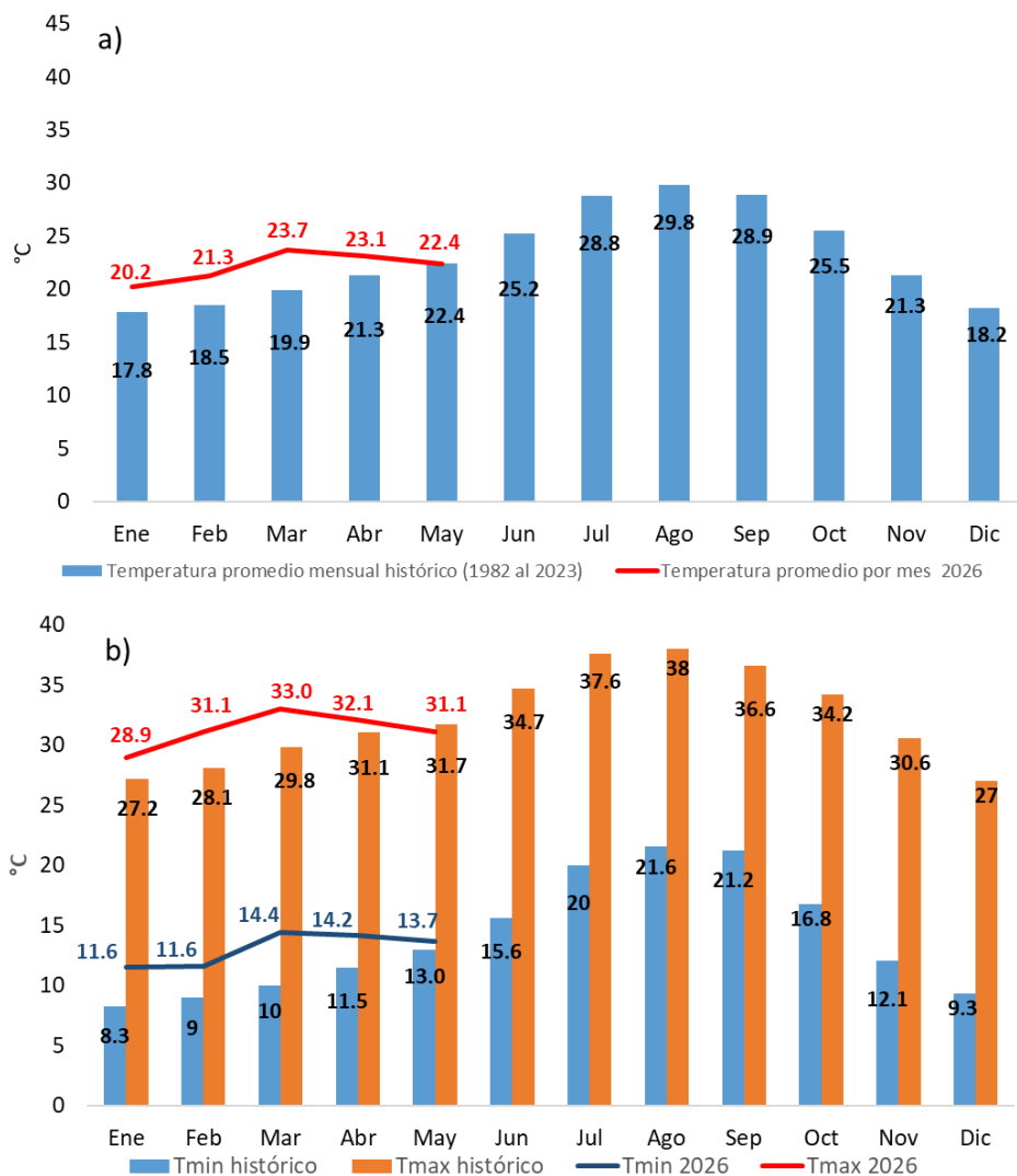
Figura 10.2: a) Comparativo de los promedios mensuales de la temperatura media (periodo 1982-2023) con respecto al registrado en el mes de mayo de 2026. b) Comparativo entre promedios de temperaturas máximas y mínimas históricas (1982-2023) con respecto a promedios presentados en el mes de mayo de 2026. Tmax= Temperatura máxima. Tmin= Temperatura mínima.
