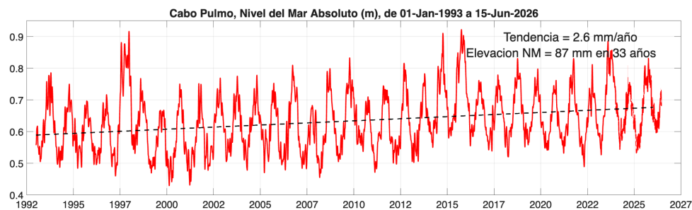
Figura 2.3: Nivel del mar absoluto (m) en Cabo Pulmo, BCS. Inicia en enero de 1993 y termina en junio de 2026. Incluye el nivel del mar con referencia al geoide y la tendencia de largo período debida al calentamiento global. Este sitio representa la variabilidad de la entrada al Golfo de California.
