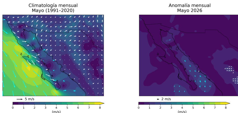
Figura 8.6: Climatología mensual y anomalía del viento superficial para mayo de 2026 a partir de productos combinados de reanálisis atmosférico. El panel izquierdo muestra la magnitud y dirección climatológica del viento a 10 m para el mes de mayo durante el periodo 1991–2020 , mientras que el panel derecho presenta la anomalía mensual correspondiente a mayo de 2026 respecto a dicha climatología. Los colores representan la magnitud del viento o de su anomalía, mientras que los vectores muestran la dirección del flujo superficial, integrando información de ERA5 sobre océano (vectores en cian) y ERA5-Land sobre superficie continental (vectores en blanco).
