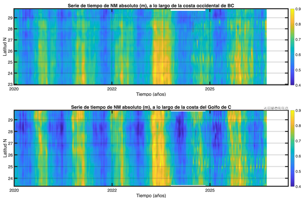
Figura 2.2: Los últimos años de la evolución del nivel del mar (NM absoluto) a lo largo de las dos costas de la península de BC desde enero de 2020 hasta junio de 2026. Arriba: costa occidental; abajo: costa del Golfo de California.
