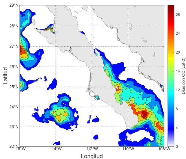
Figura 5.2: Días con ondas de calor categoría 2 en el área de estudio para mayo de 2026.
