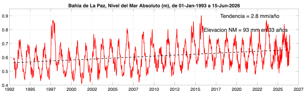
Figura 2.4: Nivel del mar absoluto (m) en la bahía de La Paz, BCS. Inicia en enero de 1993 y termina en junio de 2026. Incluye el nivel del mar con referencia al geoide y la tendencia de largo período debida al calentamiento global.
