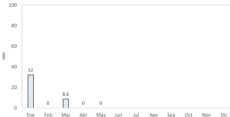
Figura 10.4: Precipitación registrada al mes de mayo de 2026.
