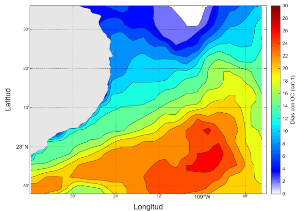
Figura 5.4: Cantidad con días con ondas de calor de categoría 1 en Cabo Pulmo y zonas aledañas para abril de 2026.
