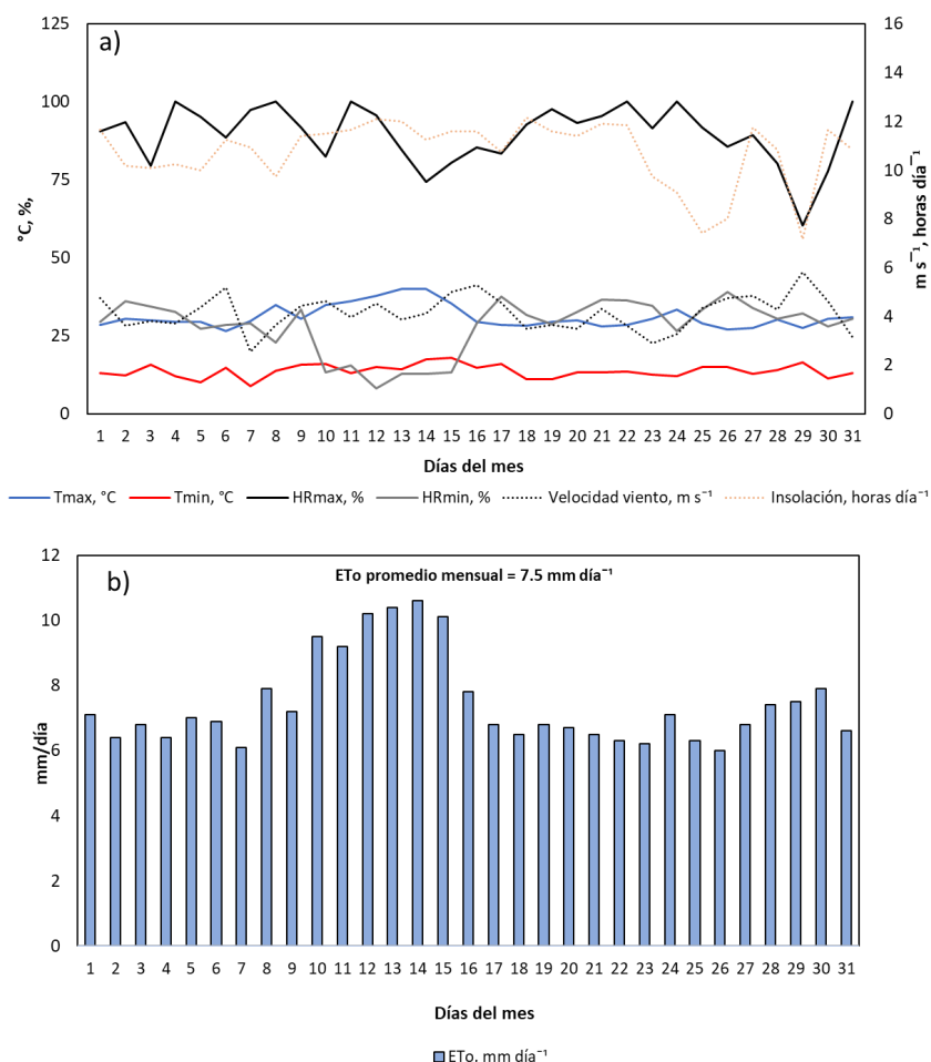
Figura 10.3: a) Comportamiento de la temperatura máxima (Tmax), temperatura mínima (Tmin), humedad relativa máxima (HRmax) y mínima (HRmin), velocidad del viento e insolación en el mes de mayo de 2026. b) Comportamiento de la evapotranspiración potencial (ETo) en el mes de mayo de 2026.
