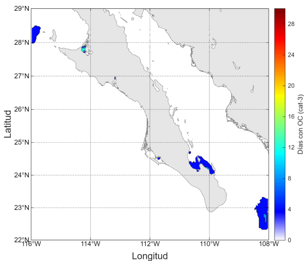
Figura 5.3: Días con ondas de calor categoría 3 en el área de estudio para mayo de 2026.
