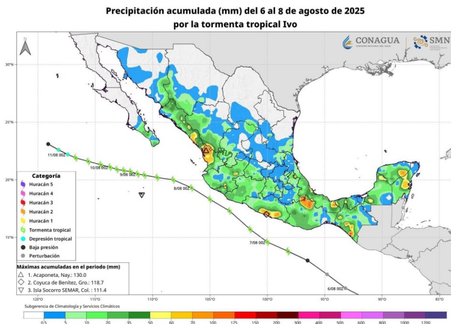
Figura 9.2: Trayectoria de la tormenta tropical Ivo que se presentó durante el mes de agosto de 2025 en el Océano Pacífico oriental. La imagen se tomó del SMN https://smn.conagua.gob.mx/tools/RESOURCES/com_mapas_lluvias/IVO-final.jpg . Contornos en color representan la lluvia acumulada (mm) en la red de estaciones del SMN.
